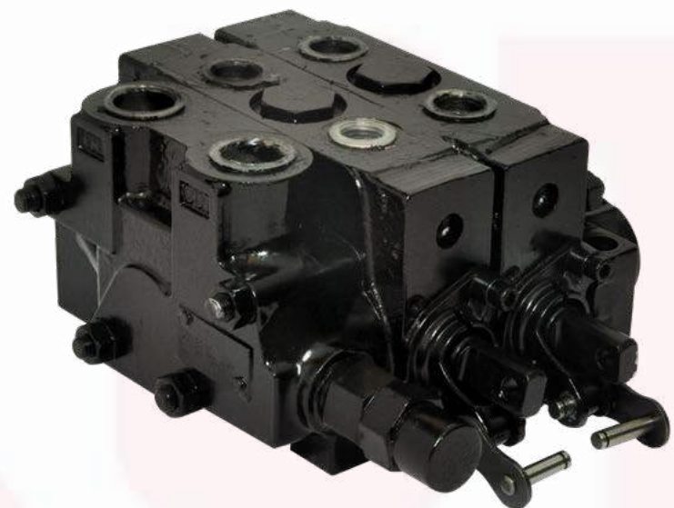
73402379 COMANDO HIDRÁULICO DUPLO V10 COM DESARME - FARMAL 80 | TL85
