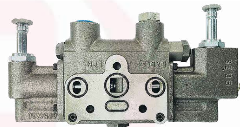
DQ44179 - CONJUNTO CORPO SUBIDA DO AUTOMATICO DA PLATAFORMA
