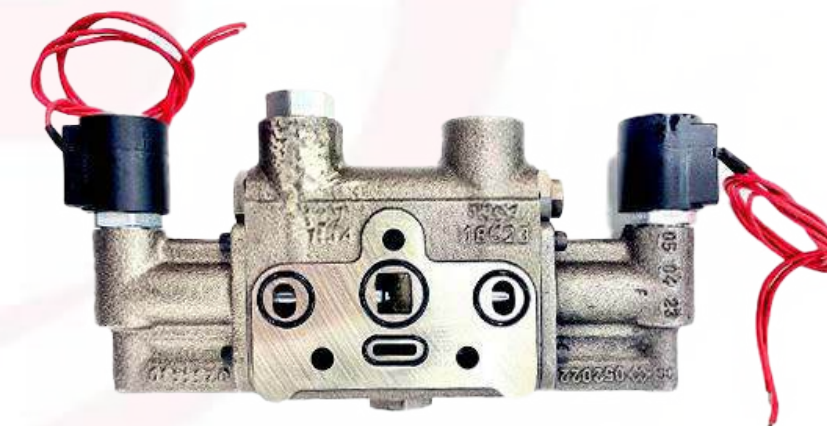
101063 FATIA SIMPLES AÇÃO COMANDO ELÉTRICO
